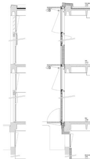
Façade avant...
